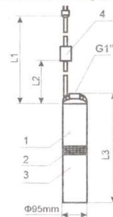
Рис. 1 Габаритные и присоединительные размеры 1 – насосная часть, 2 – фильтр, 3 – электродвигатель, 4 – конденсаторная приставка.
