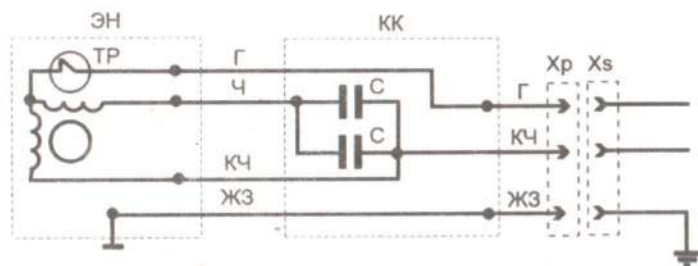
Рис 3. Схема электрическая принципиальная
