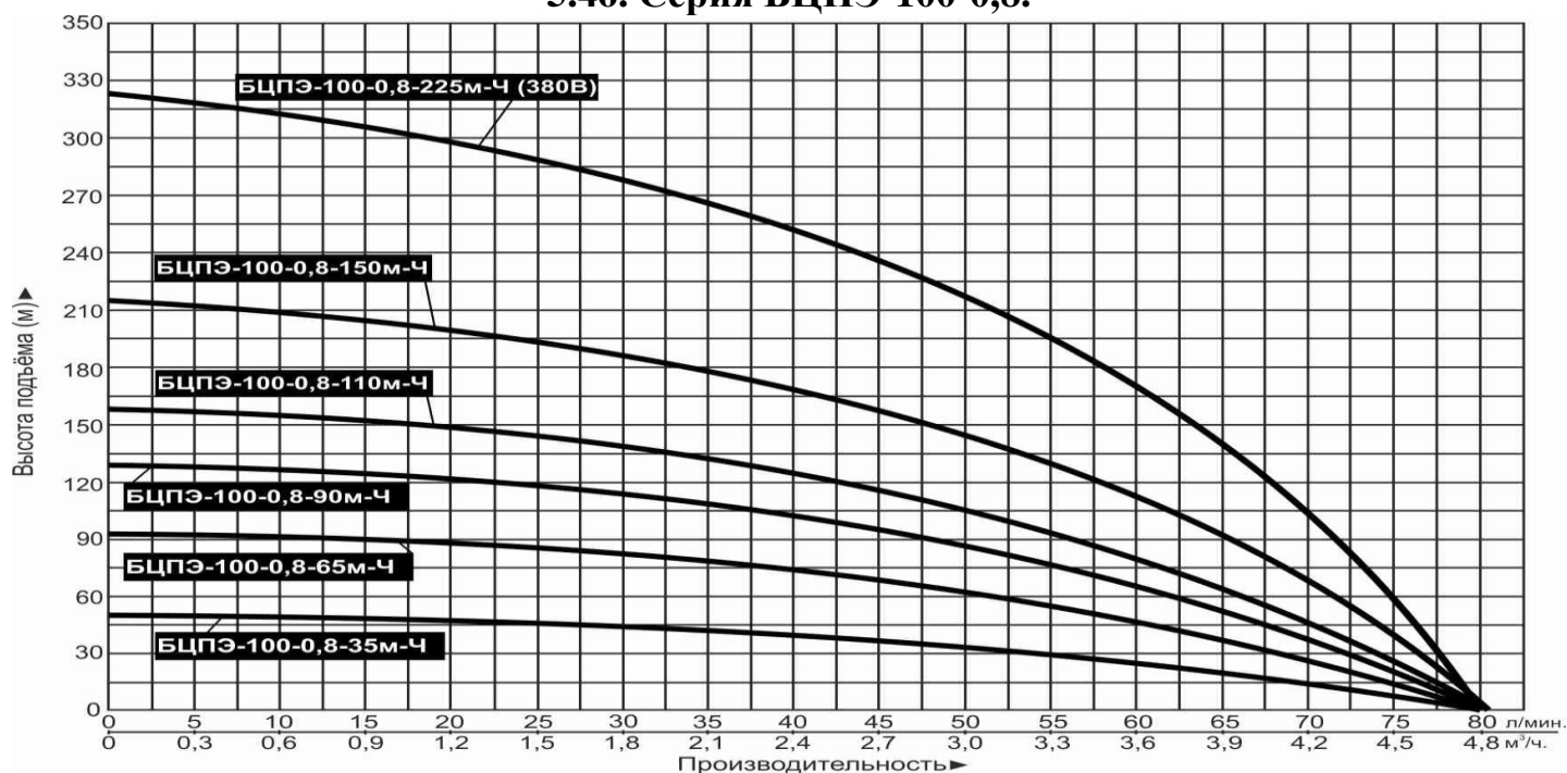
5.46. Серия БЦПЭ-100-0,8.
