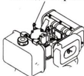
Рычаг декомпрессии
